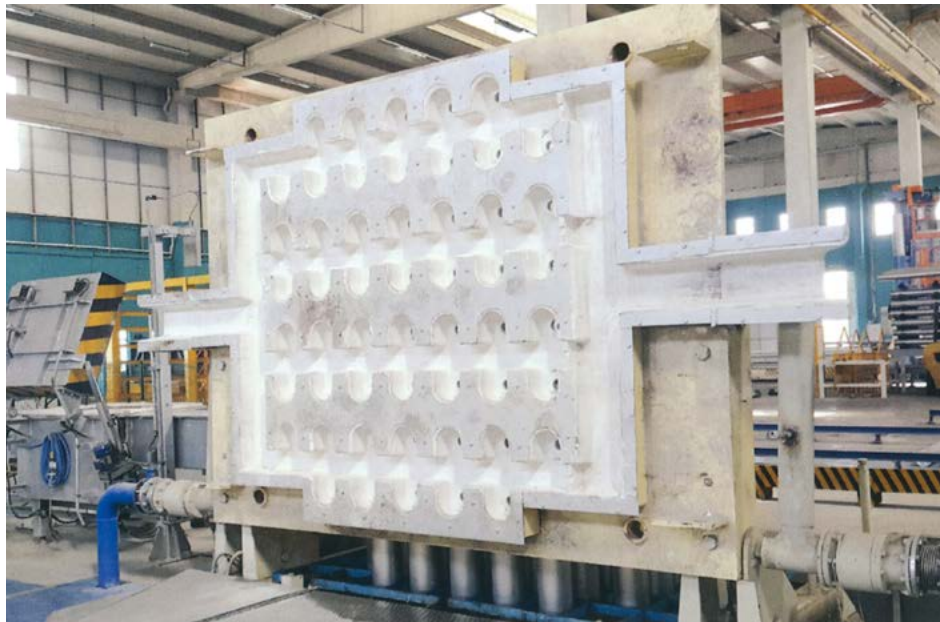
Air Slip and Hot Top Billet Casting Tables Air Slip ve Hot Top Döküm Masaları
